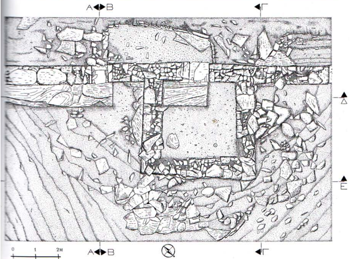
Είχ. 236γ. Ο ΒΑ. προμαχών (ὕπὸ Ἀ. Γούναρη).
