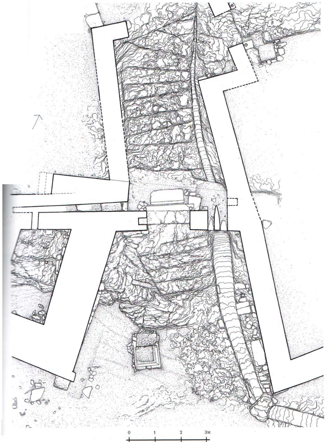
Είχ. 177β. Ἡ πύλη καὶ ἡ βαθμιδωτὴ ὁδὸς M1 (ὕπὸ Γ. Ἀντωνίου).
