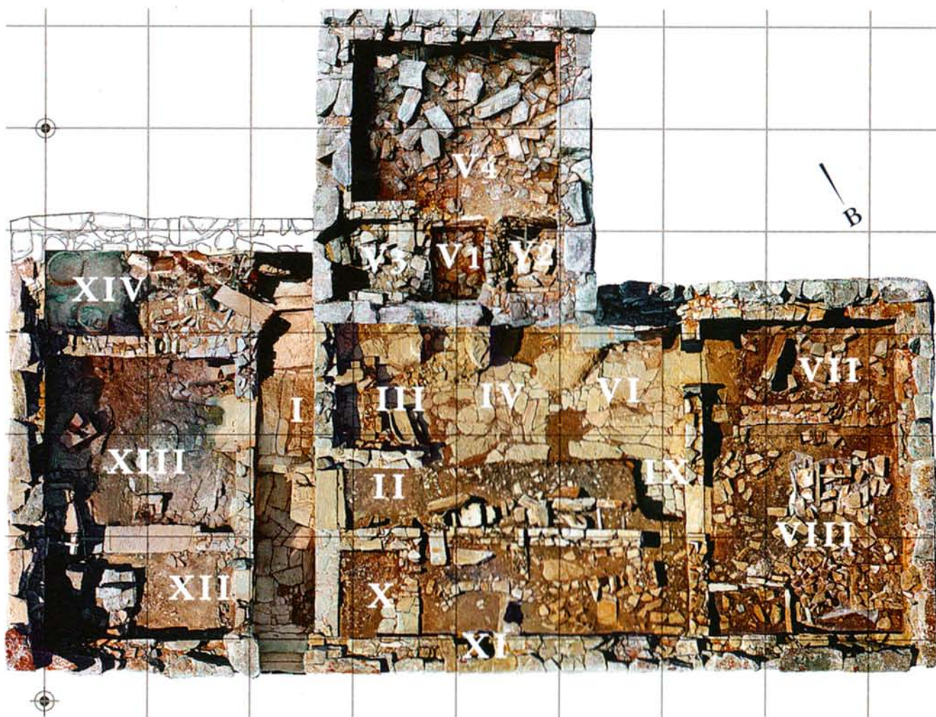
28. Φωτογραμμετρική κάτοψη του ἐσωτερικοῦ χώρου τῆς Αὐλῆς καὶ τοῦ κυρίως πύργου (Α. Χρυσάνθου, 2007).
