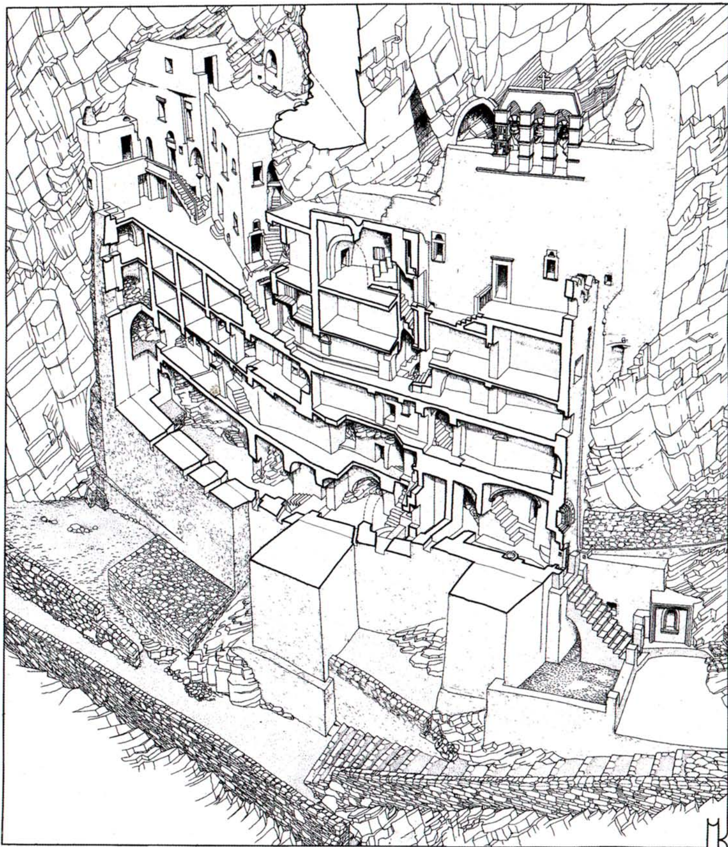
Άξονομετρική τομή του έσωτερικού τῆς Μονῆς. Σχέδιο Μανόλη Κορρέ.
